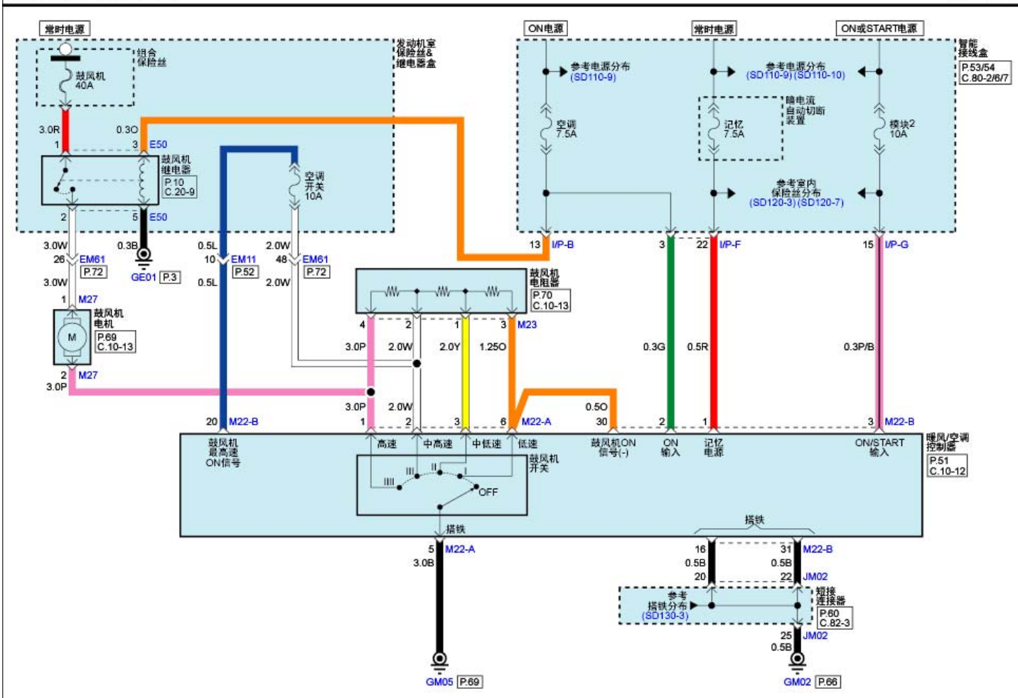
空调控制系统(手动)(1)
